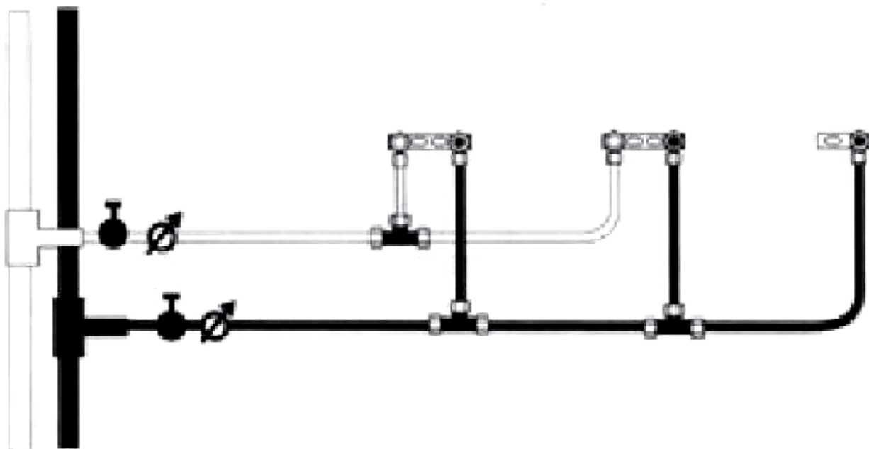
Рис2. Последовательная схема с тройниками
