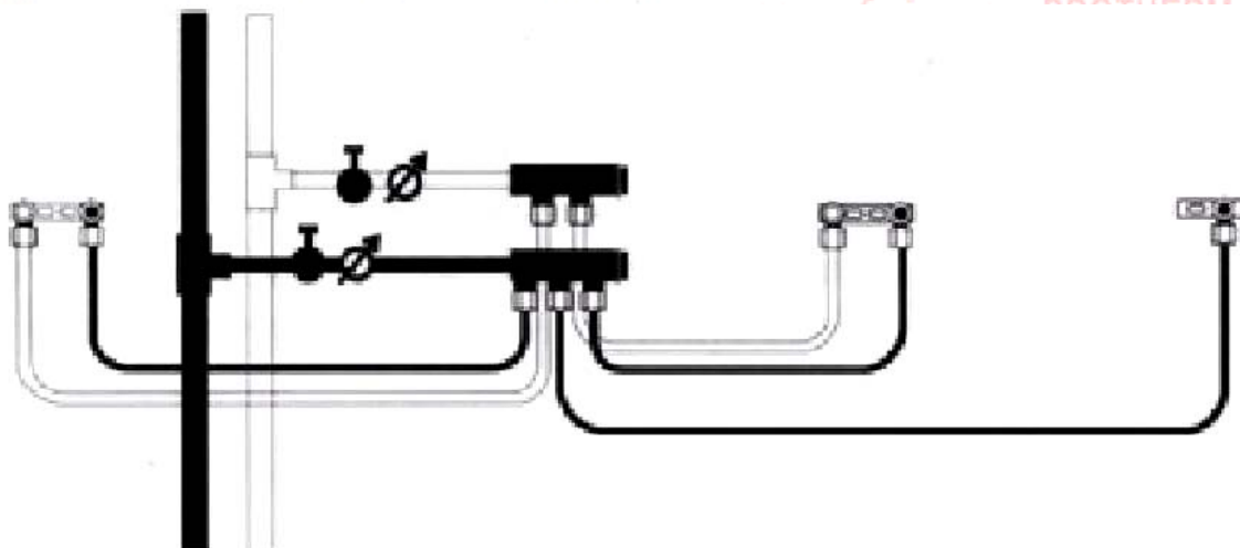
Рис 1. Коллекторная схема
