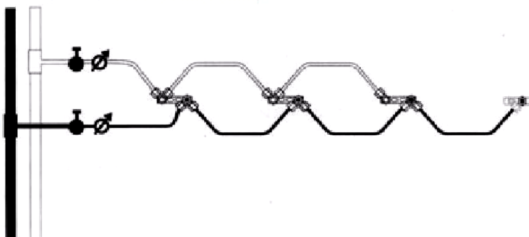
Рис.3. Последовательная схема с установочными тройниками
